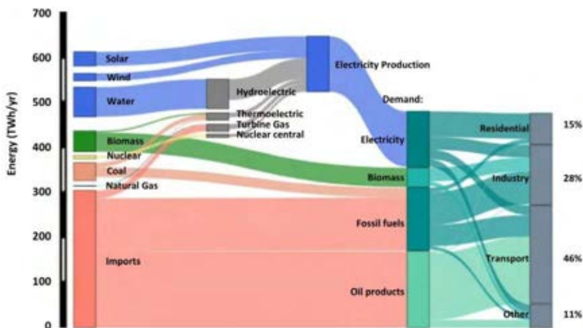
Figura 4. Diagrama de Sankey del escenario Inflexión a 2050. Fuente: Elaboración propia a partir de datos del PEN 2020-2050, U.S. Department of Energy 2.019 y Plazas-Niño 2.023.
