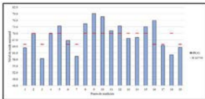
Figura 2. Niveles de ruido ambiental jornada ordinaria diurna vs el nivel máximo permisible.
