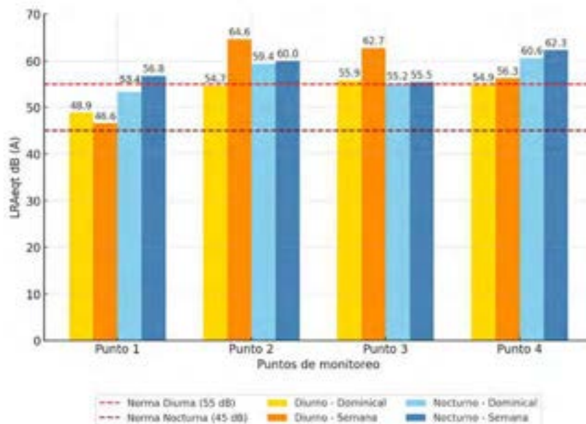
Figura 4. Resultados monitoreo de ruido ambiental horario diurno y nocturno.
