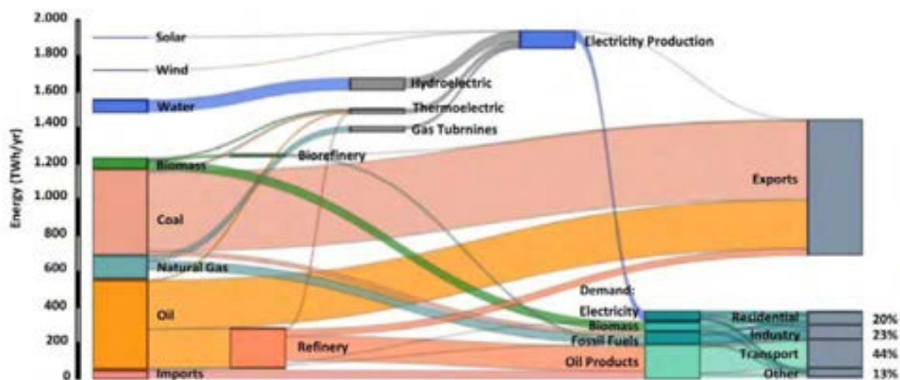
Figura 1. Diagrama de Sankey del sistema energético colombiano en 2021
