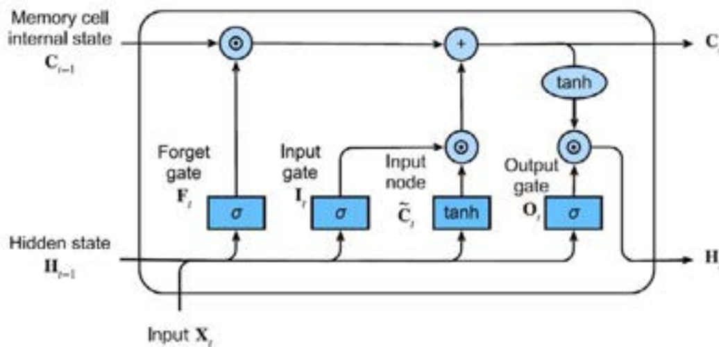
Figura 1. Esquema red LSTM () (Czum, 2020)
