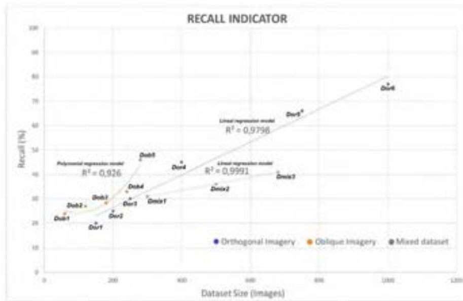
Figura 2. Resultados del indicador recall para cada dataset. Fuente: Elaboración propia.
