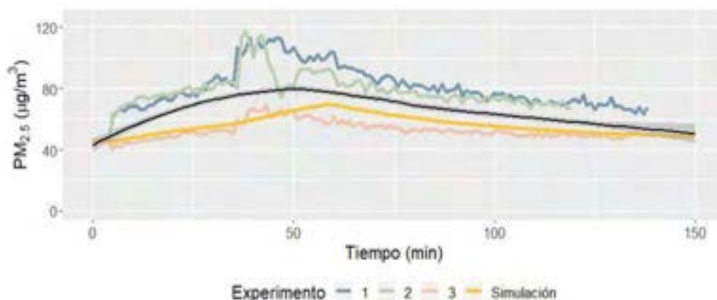
Figura 2. Comportamiento temporal de PM_{2,5} antes, durante y después del uso de velas aromática, apagadas con un trapo húmedo, en un escenario con poca o nula ventilación
