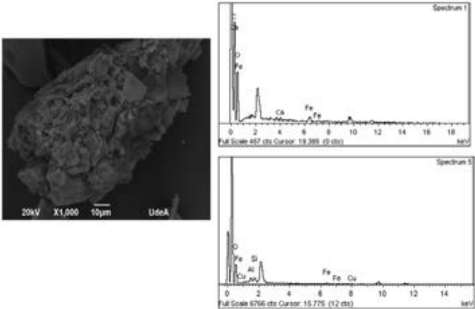
Figura 1. Análisis SEM-EDS de las nanopartículas de carbón (NP) provenientes de las minas de La Loma-Cesar. La imagen A muestra la forma irregular de las NP y, al lado el espectro composicional obtenido por EDS.
