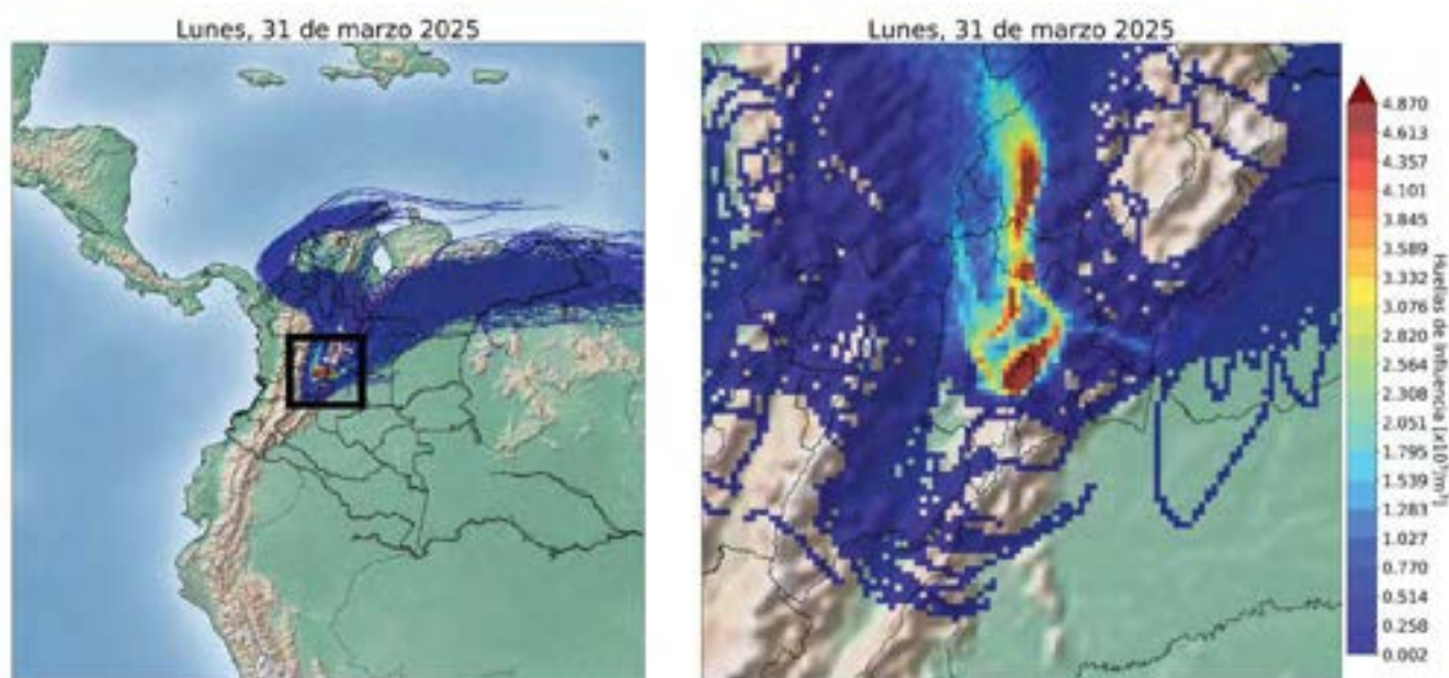
Figura 1. Huella de influencia generada a partir del modelo HySplit para el 31 de marzo del 2025 a las 8 am. Izquierda resultados de simulación con los archivos del modelo GFS y derecha salida con el modelo WRF. Fuente: Elaboración propia.
