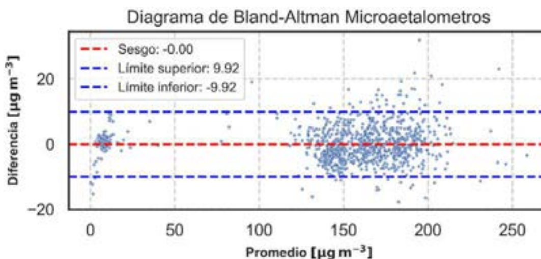
Figura 4. Diagrama de Bland-Altman para mediciones simultáneas de eBC con microaetalómetros de la misma referencia con una resolución temporal de 1 segundo. Fuente: Elaboración propia.
