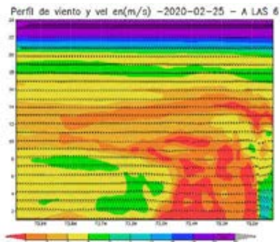
Figura 1. Perfil del viento y velocidad en m/s en un corte vertical este-oeste en el centro de la zona minera del departamento del Cesar para el 25-02-2020 a las 6.
