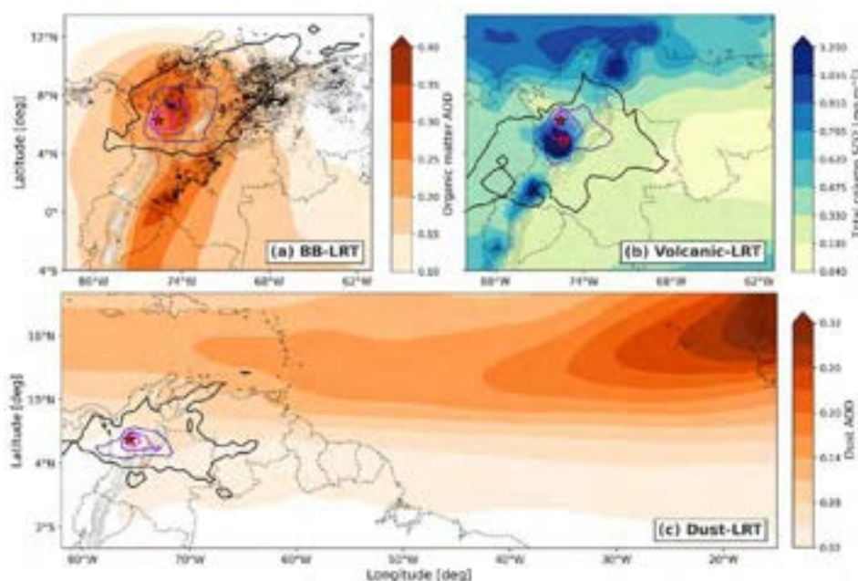
Figura 3. Distribución espacial media de (a) OM-AOD, (b) TCSO2 y (c) Du-AOD, y retrotrayectorias que llegan al VA. Los contornos encierran las regiones desde las cuales el 20%, el 10%, el 5% y el 1% de las masas de aire llegan al VA. Los puntos grises en el panel (a) indican puntos críticos según MODIS asociados con incendios (nivel de confianza del 70%). La estrella roja marca la ubicación de la VA y el círculo rojo en el panel (b) marca la ubicación del Nevado del Ruiz. Los finos contornos negros muestran la elevación del terreno de 1500 a 5000 m s.n.m. Fuente: elaboración propia.
