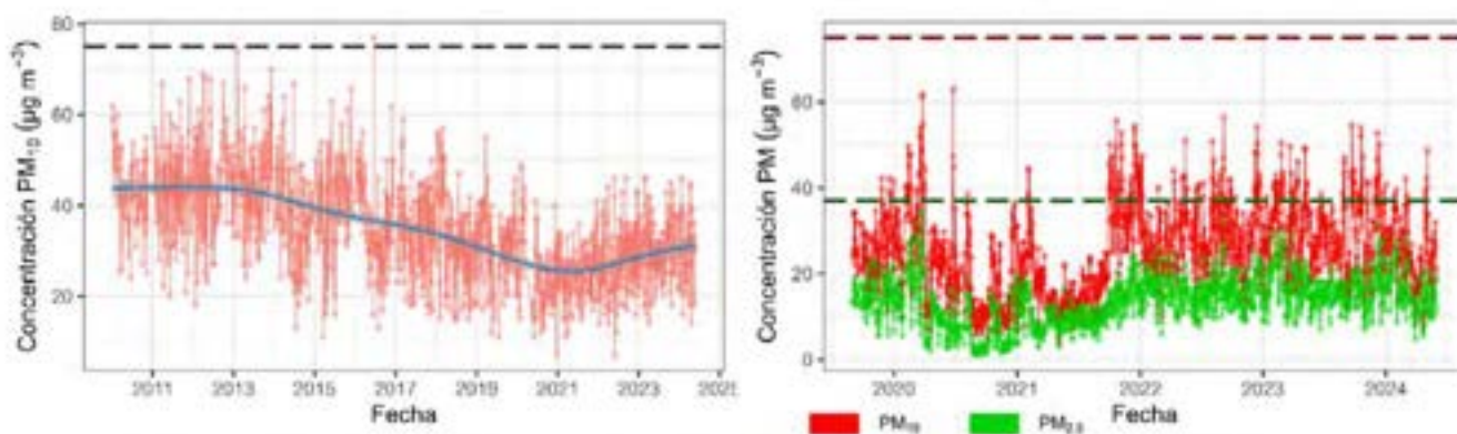
Figura 3. Variación histórica de concentraciones diarias de PM_{10} y PM_{2.5} en la estación Liceo para equipos manual (izquierda) y automático (derecha). la línea punteada indica el límite normativo definido en la Resolución 2254 de 2017. Fuente: propia
