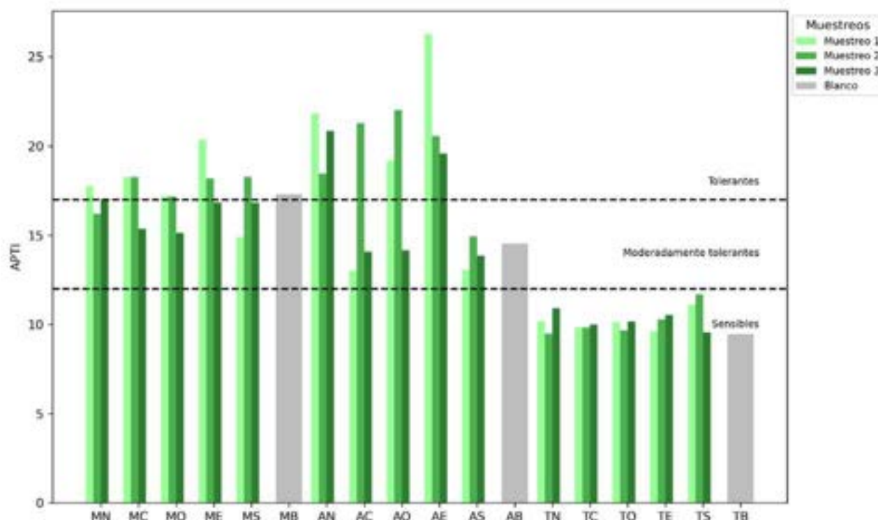
Figura 2. Valores APTI de las especies evaluadas. Fuente: elaboración propia.
