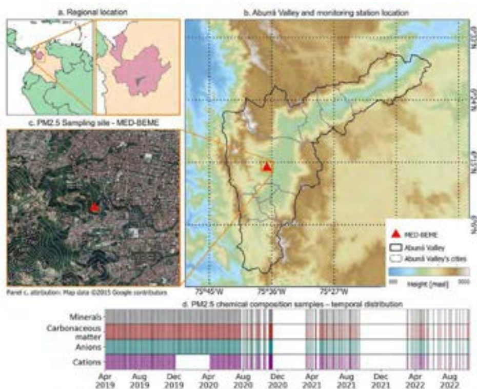
Figura 1. (a) Ubicación y (b) Geomorfología del VA con los 10 municipios (líneas grises discontinuas); (c) Ubicación de la estación de campaña de muestreo de PM_{2.5} (MED-BEME) en triángulo rojo en los paneles (b) y (c), y (d) Cobertura temporal de la campaña de muestreo de PM_{2.5} . Fuente: elaboración propia.
