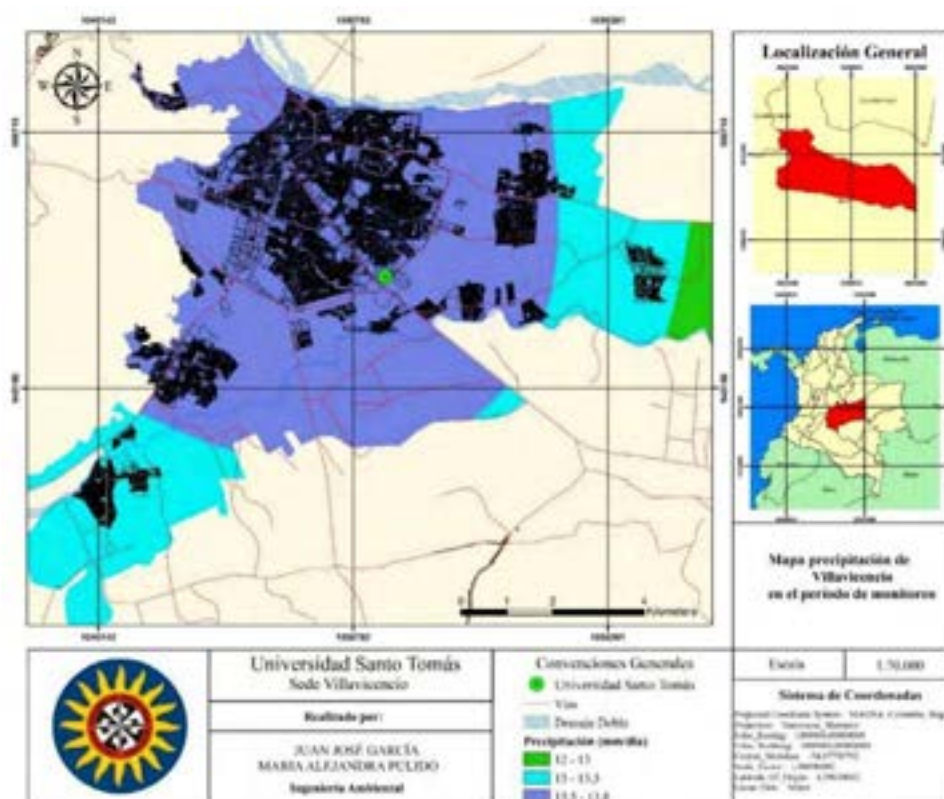
Mapa precipitación
