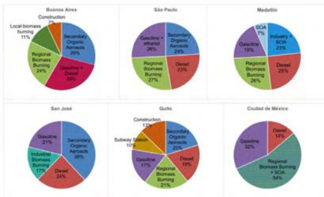
Figura 2. Contribución de las distintas fuentes al carbono total según la modelización PMF para las seis ciudades de este estudio.
