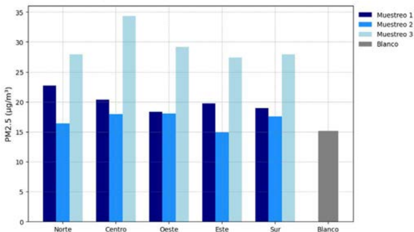
Figura 3. Concentración ambiental de PM2.5 . Fuente: elaboración propia.
