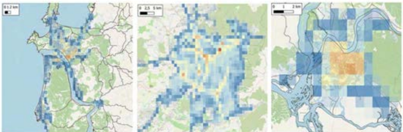
Figura 1. Desagregación espacial de emisiones para Concepción, Santiago y Valdivia en el año 2020. Fuente [1]
