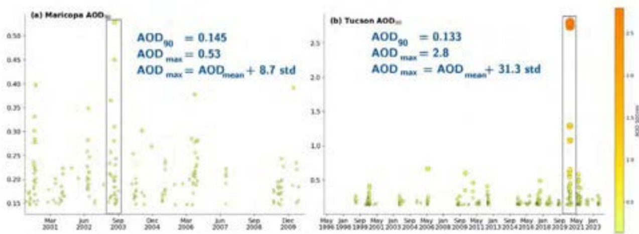
Figura 1. Eventos extremos en las estaciones de a) Maricopa en Junio del 2003 y b) Tucson en Septiembre del 2020. Fuente: Elaboración propia.
