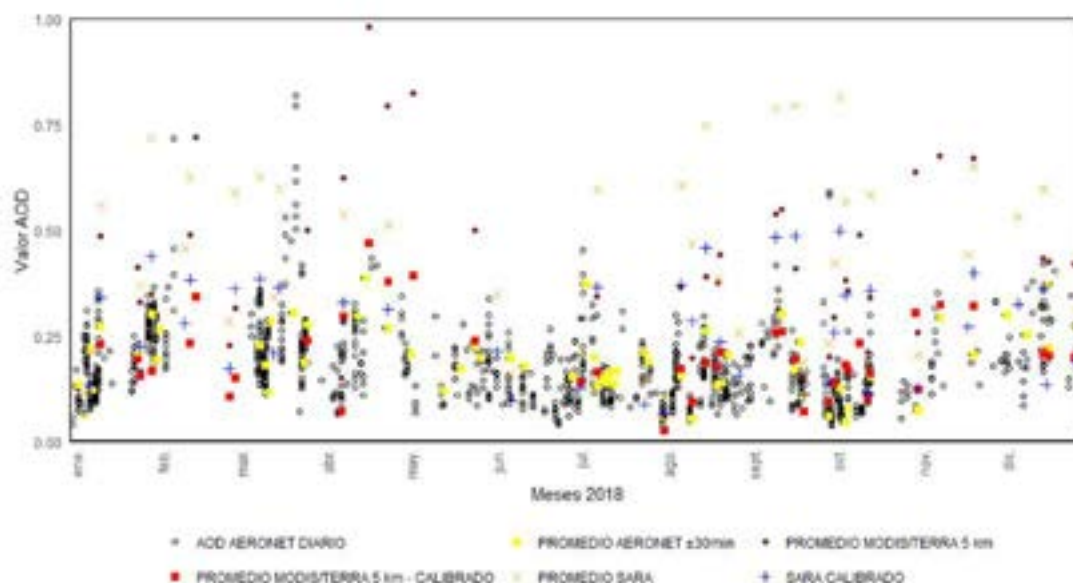
Figura 2. Resultados y calibración de AOD en SARA y MODIS . Fuente: Elaboración propia.
