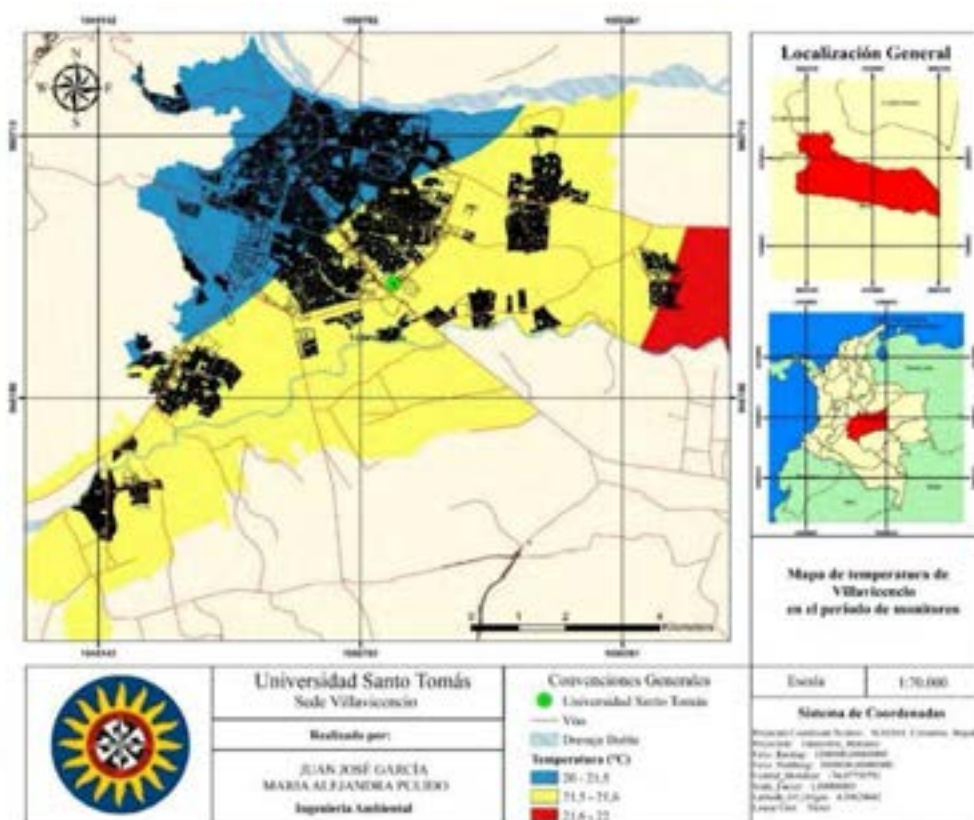
Mapa temperatura
