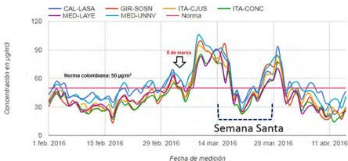
Figura 2. Concentraciones diarias de PM_{2.5} registradas en las estaciones automáticas de la Red de monitoreo de calidad del aire del Valle de Aburrá. Fuente: Área Metropolitana del Valle de Aburrá, Universidad Pontificia Bolivariana, Convenio 335 de 2016.
