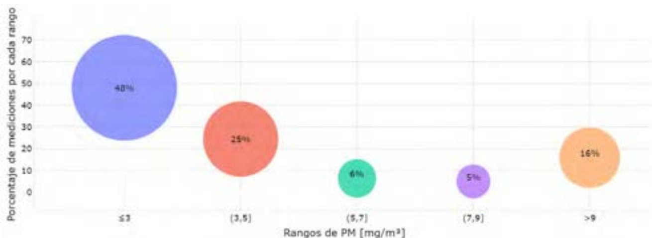
Figura 4. Distribución de los resultados respecto a rangos de PM. Fuente: Elaboración propia.
