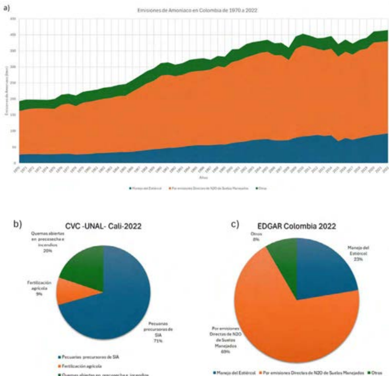
Figura 2. a) Emisiones de \text{NH}_3 Colombia 1970-2022-EDGAR. b) Inventarios de emisiones de amoníaco Corporación Autónoma Regional del Valle del Cauca (CVC) y Universidad Nacional de Colombia c) Emisiones de amoníaco EDGAR-2022. Fuente: Elaboración propia (Rueda Saa et al., 2022, European Commission [EDGAR], 2023).
