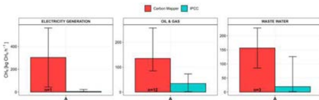
Figura 5. Comparación del flujo de CH 4 entre la campaña colombiana Carbon Mapper y las metodologías del IPCC. "n" representa el número de columnas identificadas. Fuente: Elaboración propia
