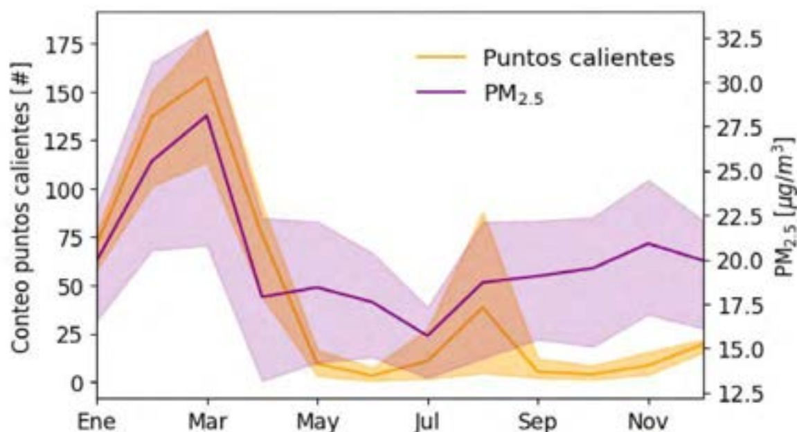
Figura 2. Ciclo anual del conteo de puntos calientes y concentración del PM_{2.5} . Sombreado el rango intercuartil IQR. Fuente: elaboración propia.
