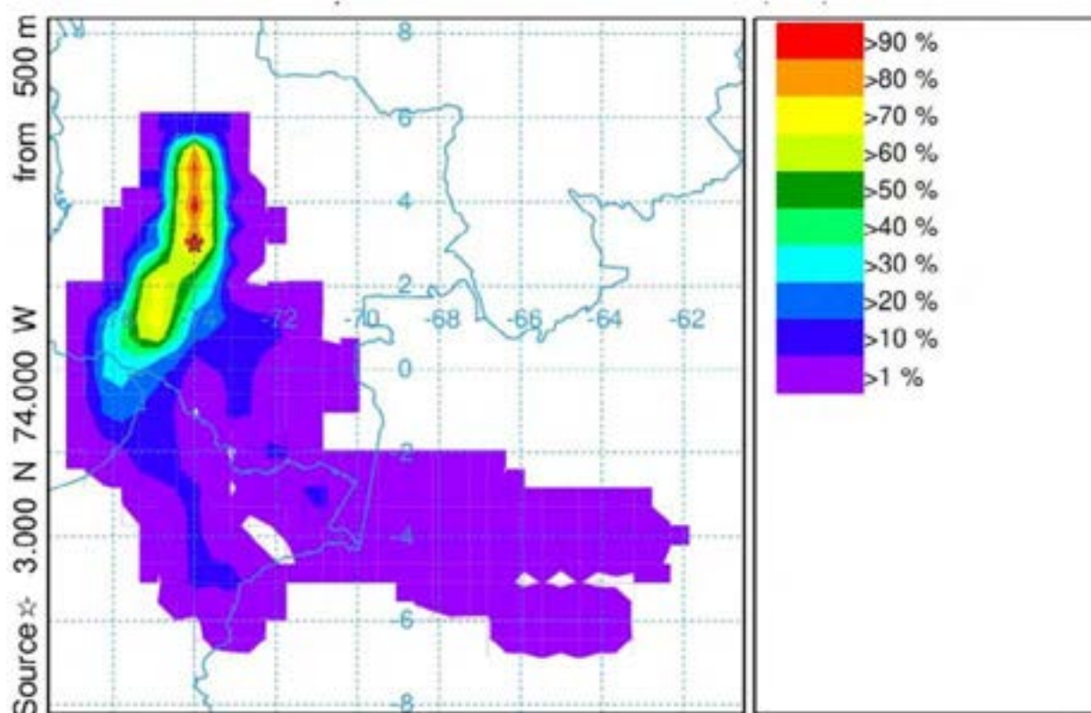
Figura 3. Retrotrayectoria probabilística de una parcela de aire que llegó a Bogotá el 4 de septiembre de 2024 a partir de información del modelo GFS. Fuente: HYSPLIT-NOAA
