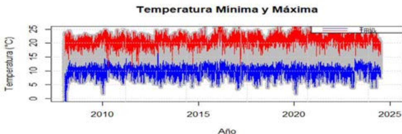
Figura 2. Temperatura máxima 2008-2024 Estación de Alto Rendimiento. Fuente: Elaboración propia.
