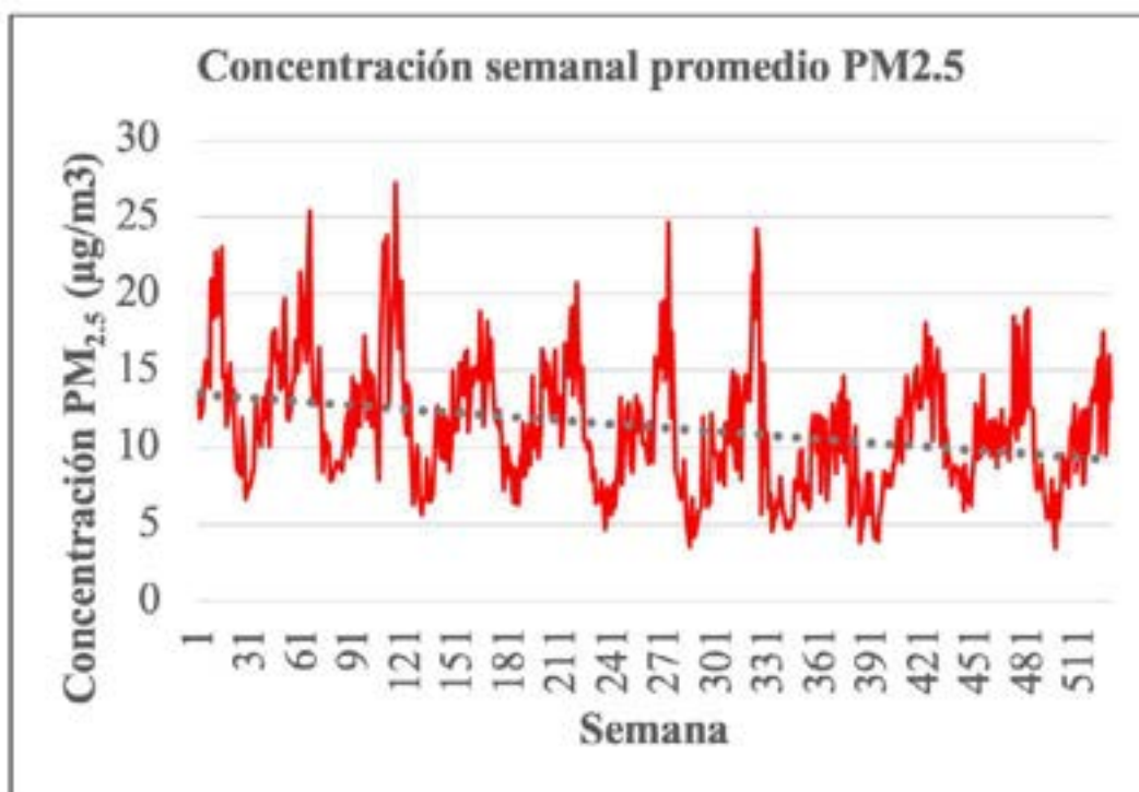
Figura 3. Concentración semanal promedio de PM 2.5 cuadrante Noroccidente años 2014-2024. Fuente: Elaboración propia.
