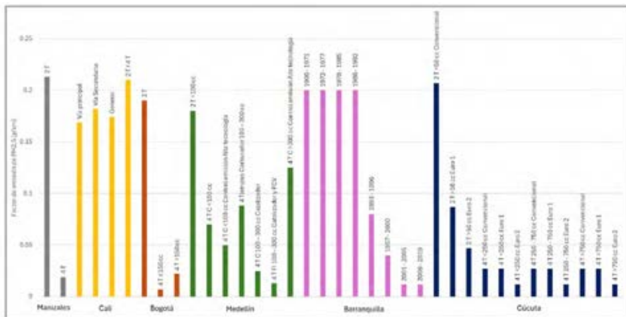
Figura 1. Comparación de factores de emisión utilizados en Colombia para la estimación de inventarios locales de emisiones.
