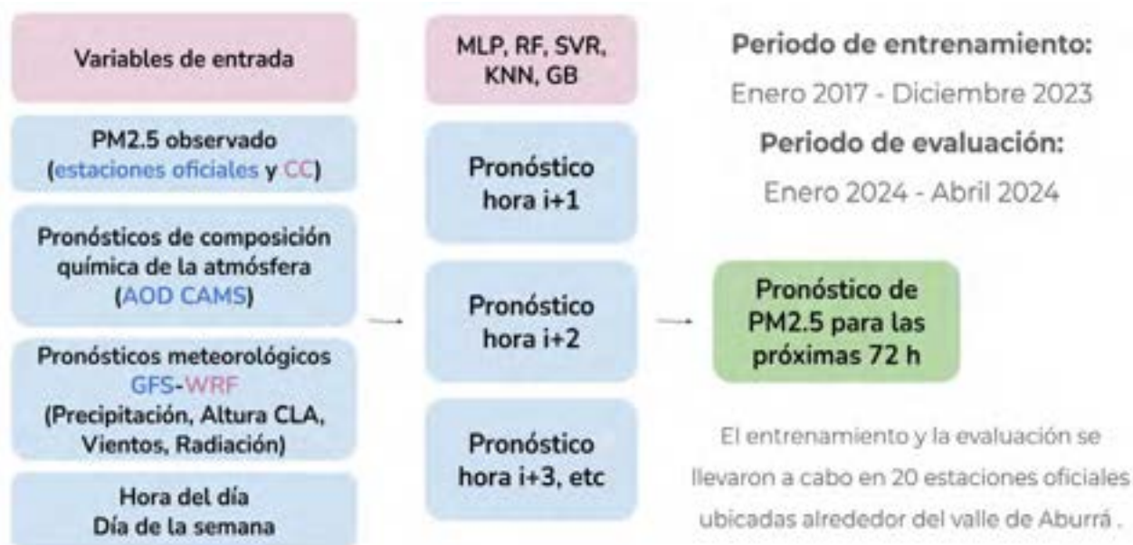
Figura 1. Esquema del sistema de pronóstico estadístico de PM2.5 para el Valle de Aburrá, mostrando las variables de entrada, los algoritmos de Machine Learning implementados, la estrategia de pronóstico por horizonte y los períodos de entrenamiento (2017-2023) y evaluación (2024).
