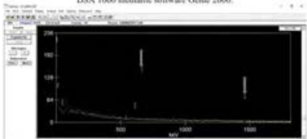
Espectro de H4 señalizando detección de Cs-137 y K-40. Espectro obtenido en interfaz Gamma digital DSA 1000 mediante software Genie 2000.
