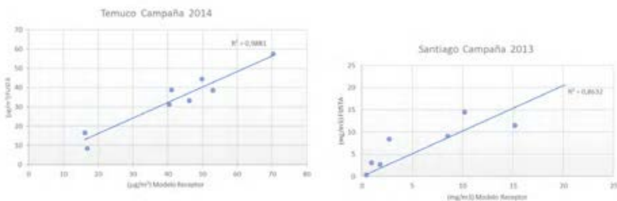
Figura 2. Correlación entre los resultados de modelo receptor campaña Temuco 2014 y Santiago 2013 y resultados algoritmo FUSTA.
