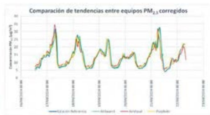
Figura 2. Comparación de tendencias para PM2.5 entre equipos corregidos.
