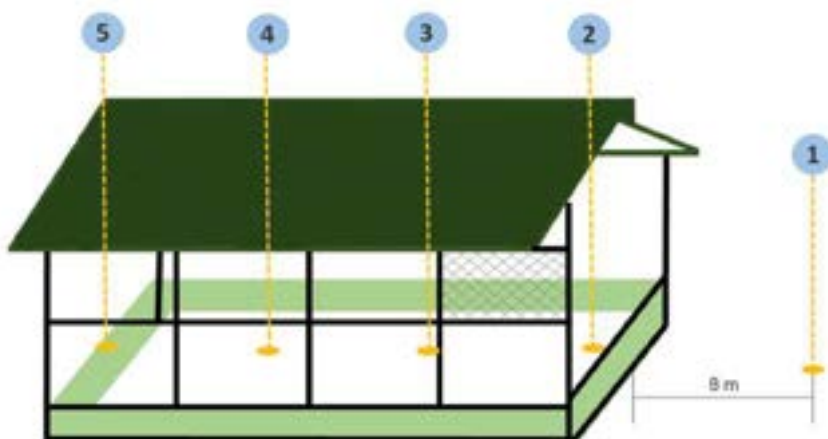
Figura 2. Ubicación de los puntos a lo largo del galpón en la campaña A. Fuente: Elaboración propia.
