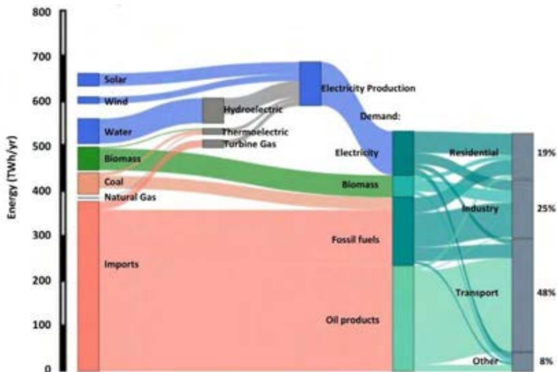
Figura 2. Diagrama de Sankey del escenario Actualización a 2050. Fuente: Elaboración propia a partir de datos del PEN 2020-2050, U.S. Department of Energy 2.019 y Plazas-Niño 2.023.
