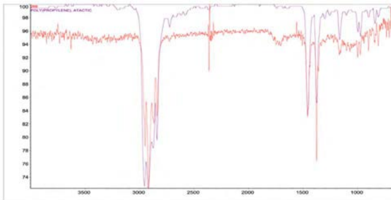
Figura 5. Espectro FTIR partícula de polipropileno
