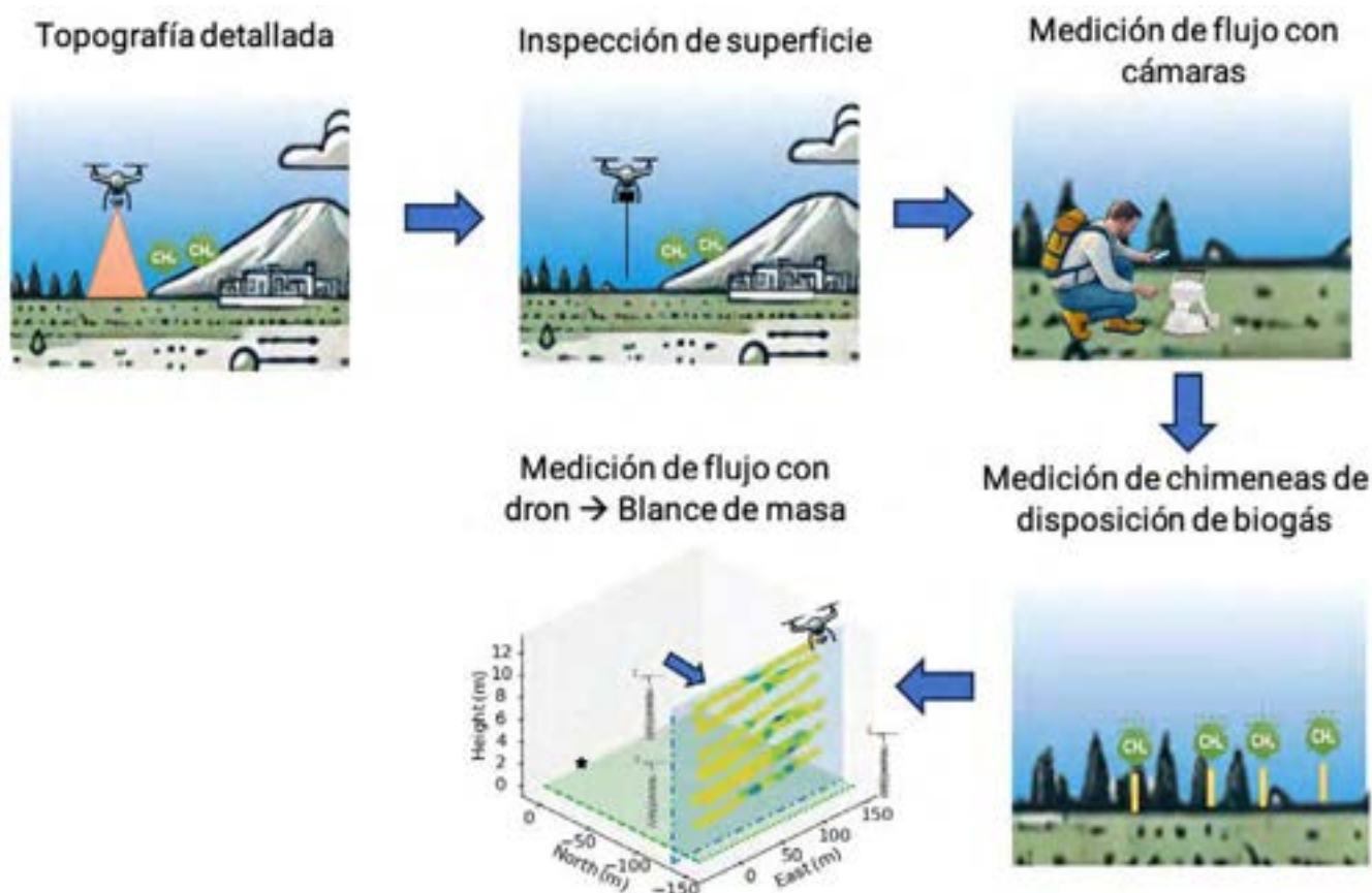
Figura 1 Ejemplo de la estrategia metodológica diseñada para la caracterización y cuantificación de las emisiones en rellenos sanitarios. Fuente: Elaboración propia.
