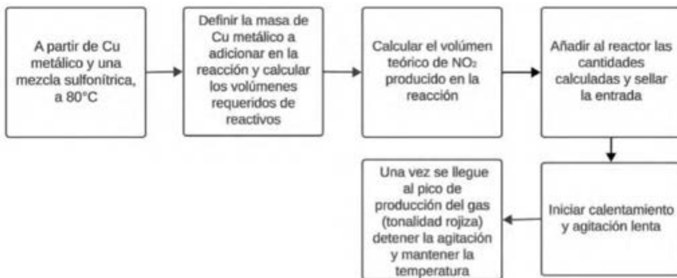
Figura 2. Puesta en marcha columna; proceso de producción NO2 y SO2. Fuente: Autoría propia, 2025.
