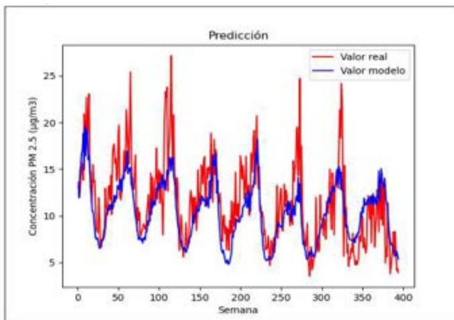
Figura 6. Predicción de concentración semanal con datos de entrenamiento cuadrante noroccidente. Fuente: Elaboración propia.ia.
