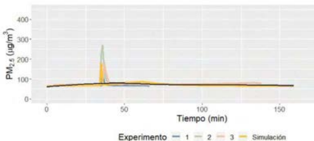
Figura 4. Comportamiento temporal de PM 2,5 antes, durante y después del uso de velas aromática, apagadas con un trapo húmedo, en un escenario con ventilación u \geq 0,5 \frac{m}{s}
