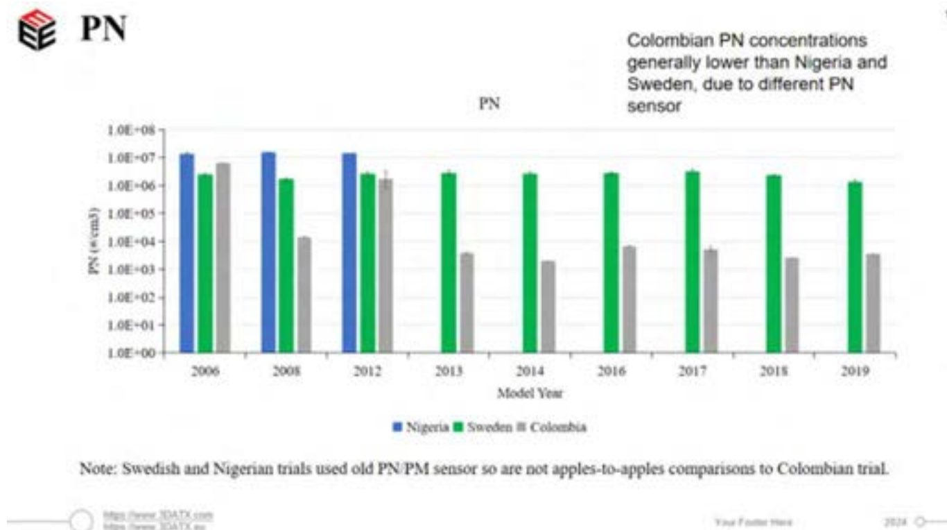
Grafica 2. Comparativo de concentraciones de Numero de partículas en las pruebas en Colombia, frente a pruebas en Nigeria y Suecia.
