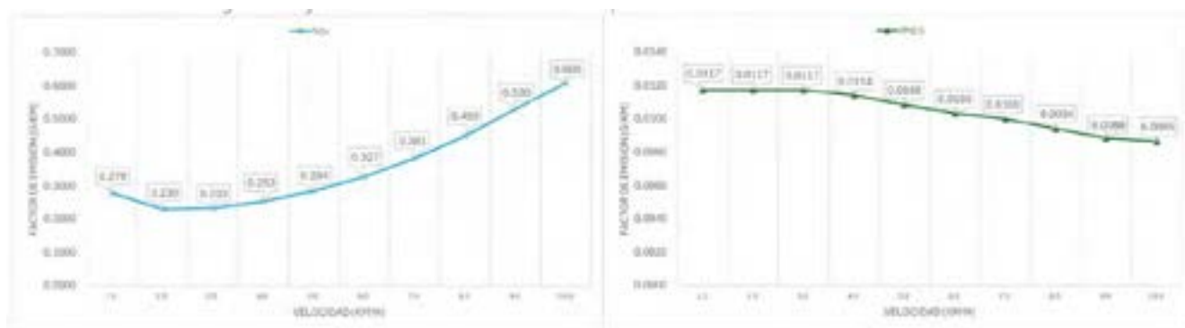
Figura 2. Influencia de la velocidad en los FE para motocicletas Euro 2 menores a 250cc.
