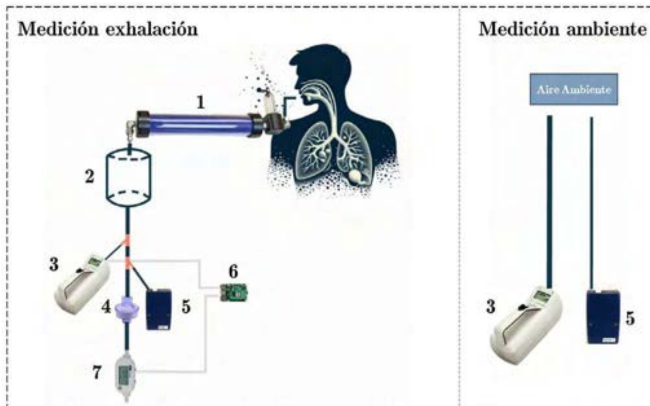
Figura 1. Montaje experimental del sistema para la medición de partículas ultrafinas y eBC. (A) Configuración del sistema para medición de concentraciones de eBC y UFP de aire exhalado. (B) Configuración del sistema para medición de concentraciones de eBC y UFP del aire inhalado (ambiente). Los componentes numerados corresponden a: (1) Desecador por difusión, (2) Cámara de retención, (3) Contador de partículas de condensación – CPC 3007, (4) Filtro de partículas, (5) MicroAeth Modelo AE51, (6) Microcomputador, y (7) Medidor de flujo másico modelo 4045.
