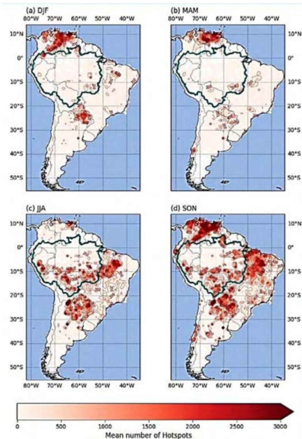
Figura 1. Distribución estacional promedio de puntos calientes en Sudamérica (2013-2023) a partir de datos satelitales MODIS
