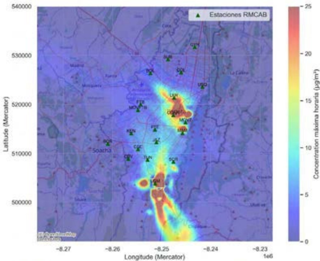
Figura 2. Distribución espacial del aporte en concentración máxima de \text{PM}_{2.5} para el periodo 10-ene a 26 feb. Fuente: Elaboración propia.
