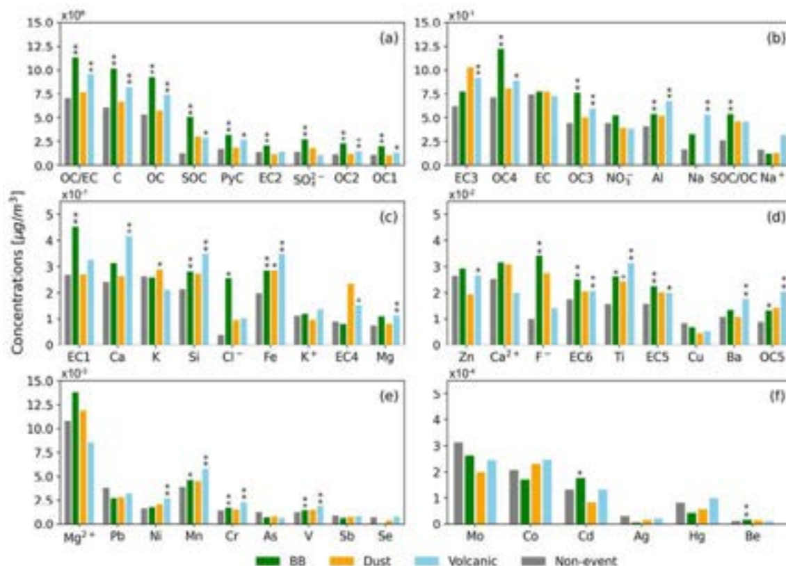
Figura 4. Concentraciones promedio de campaña con respecto a BB-LRT, Dust-LRT y Volcanic-LRT para los días de evento y no-evento. Las barras representan las concentraciones de los compuestos, con niveles de significancia en comparación con los días anteriores y posteriores a los eventos indicados como \leq 0,1 (*) o \leq 0,05 (**). El eje y varía para cada figura para resaltar mejor las concentraciones.
