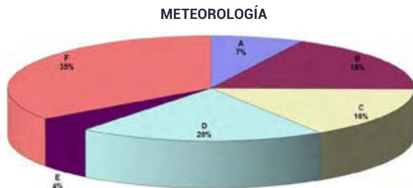
Figura 5. Estabilidad atmosférica – WRF 2023 Fuente: EYC GLOBAL 2024
