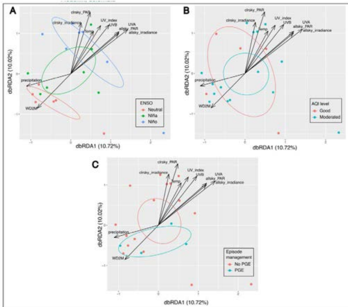
Figura 2. Ordinación de las comunidades bacterianas empleando distancia Aitchison y evaluando los efectos de (A) la temporada climática, (B) el índice de calidad del aire y (C) y el periodo de gestión de episodios. La elipse representa la distancia euclidiana al centroide del grupo, con un intervalo de confianza del 95%. Las flechas representan los gradientes de las variables ambientales continuas correlacionadas con los factores evaluados. El número de cada eje corresponde al porcentaje de la varianza explicada por las variables que restringieron el análisis.
