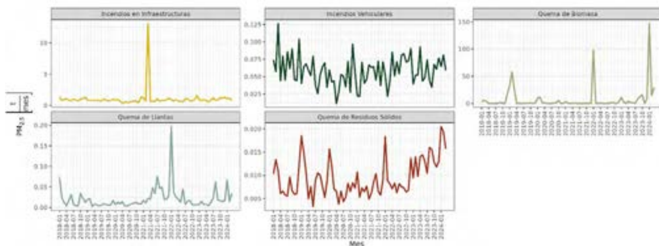
Figura 1. Emisiones mensuales de PM 2.5 por incendios y quemas a cielo abierto en Bogotá. Fuente: Elaboración propia.
