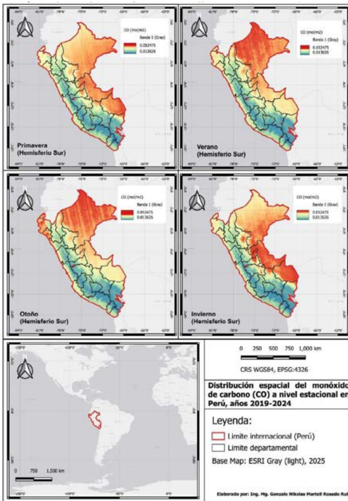
Figura 8. Mapas del comportamiento espacial del CO en el Perú, promedios estacionales en mol/m 2 , 2019 al 2024
