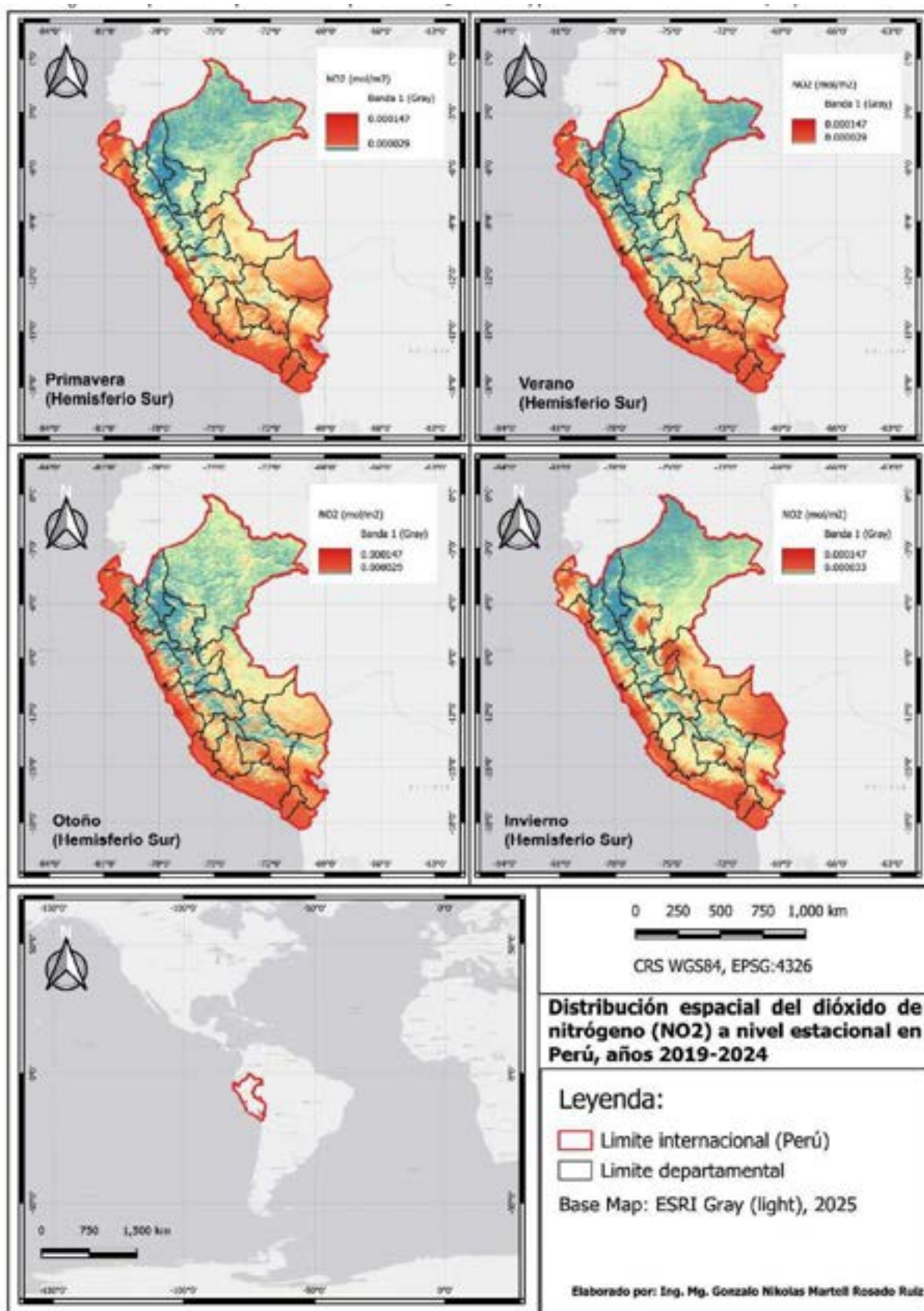
Figura 7. Mapas del comportamiento espacial del NO 2 en el Perú, promedios estacionales en mol/m 3 , 2019 al 2024
