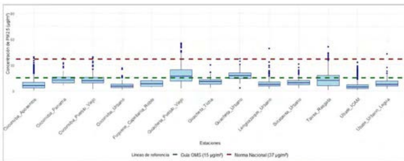
Figura 1. Promedio diario de PM_{2.5} . Fuente: Elaboración propia
