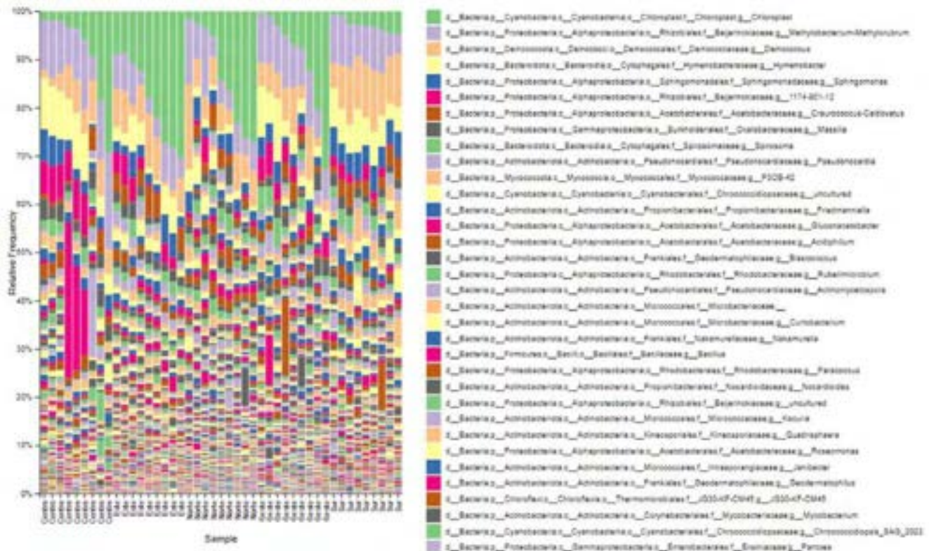
Figura 1. Frecuencia relativa de géneros bacterianos por punto de muestreo a lo largo del tiempo.
