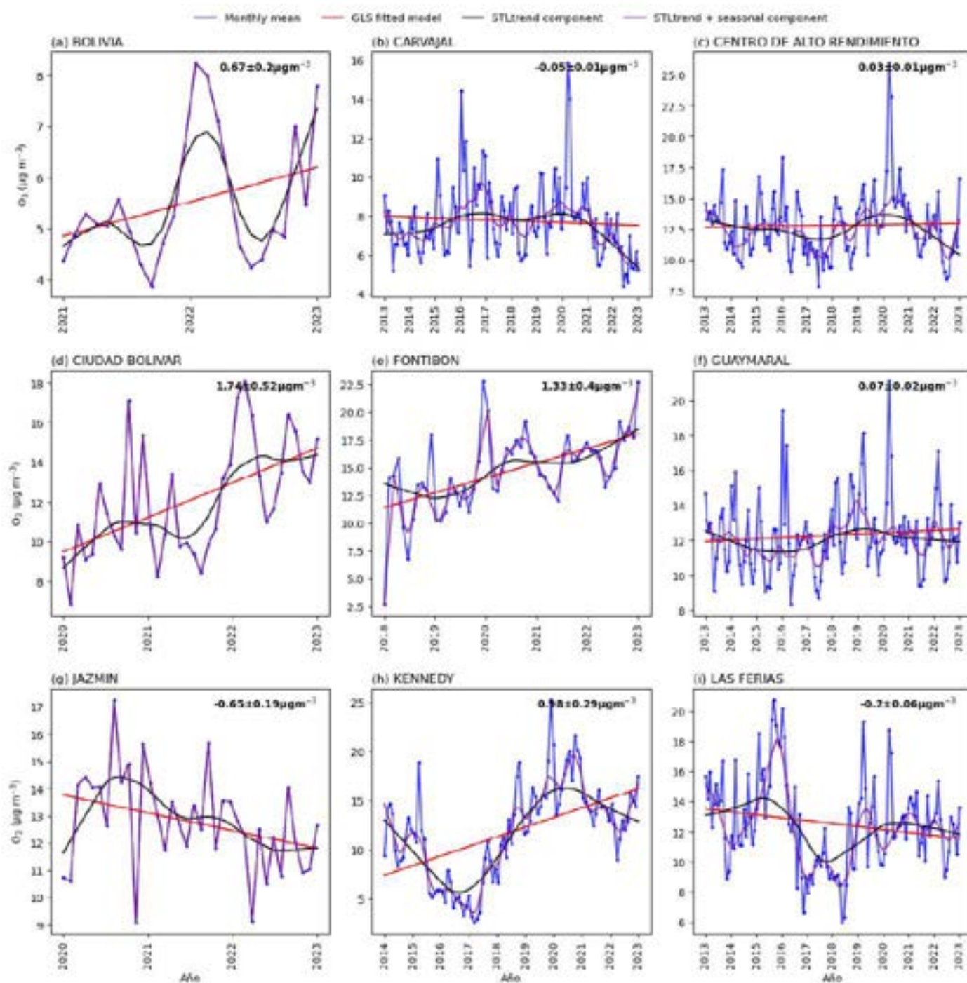
Figura 1. Análisis de Tendencia Multianual Ozono en nueve estaciones de la Red de Monitoreo de Calidad del Aire de Bogotá - RMCA. Fuente: Elaboración propia.
