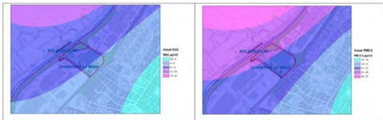
Figura 1. Resultados interpolación niveles de Calidad de aire (NO2, PM2.5).
