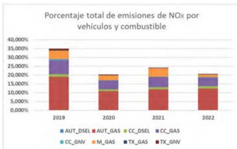
Figura.3. Evolución de las emisiones de NOx en los años 2019, 2020, 2021 y 2022, categorizada por tipo de vehículos y combustible. Fuente: Autor, 2024
