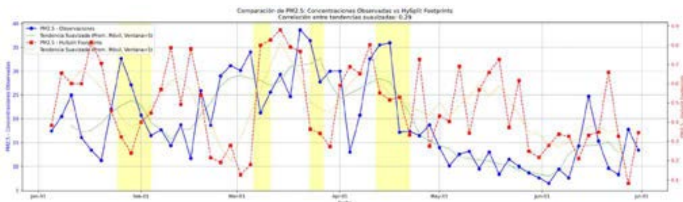
Figura 3. Serie temporal de comparación del promedio de las concentraciones de PM 2.5 de las 19 estaciones de monitoreo de RMCAB (azul) y el avance temporal de la serie del indicador de impacto (rojo). Las franjas amarillas representan los periodos en los que se declaró alerta ambiental debido a la calidad del aire en Bogotá, D.C.
