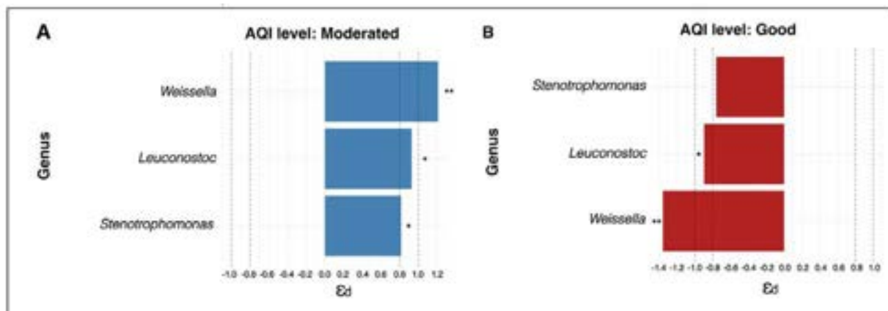
Figura 3. Resultados abundancia diferencial (ALDEx2) para índice de calidad del aire (AQI) moderado (A) y bueno (B). El eje x corresponde al tamaño del efecto. Fuente: elaboración propia.
