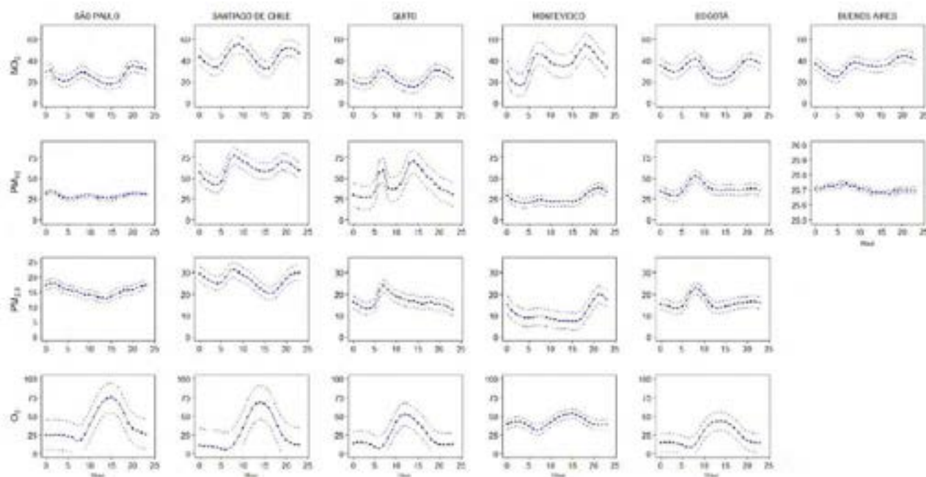
Figura 1. Promedio Horario de NO 2 (dióxido de nitrógeno), O 3 (ozono troposférico), PM 10 (material particulado de 10 micras) y PM 2.5 (material particulado de 2.5 micras) en Bogotá, Buenos Aires, Quito, São Paulo, Montevideo y Santiago de Chile, entre 2013 y 2023.
