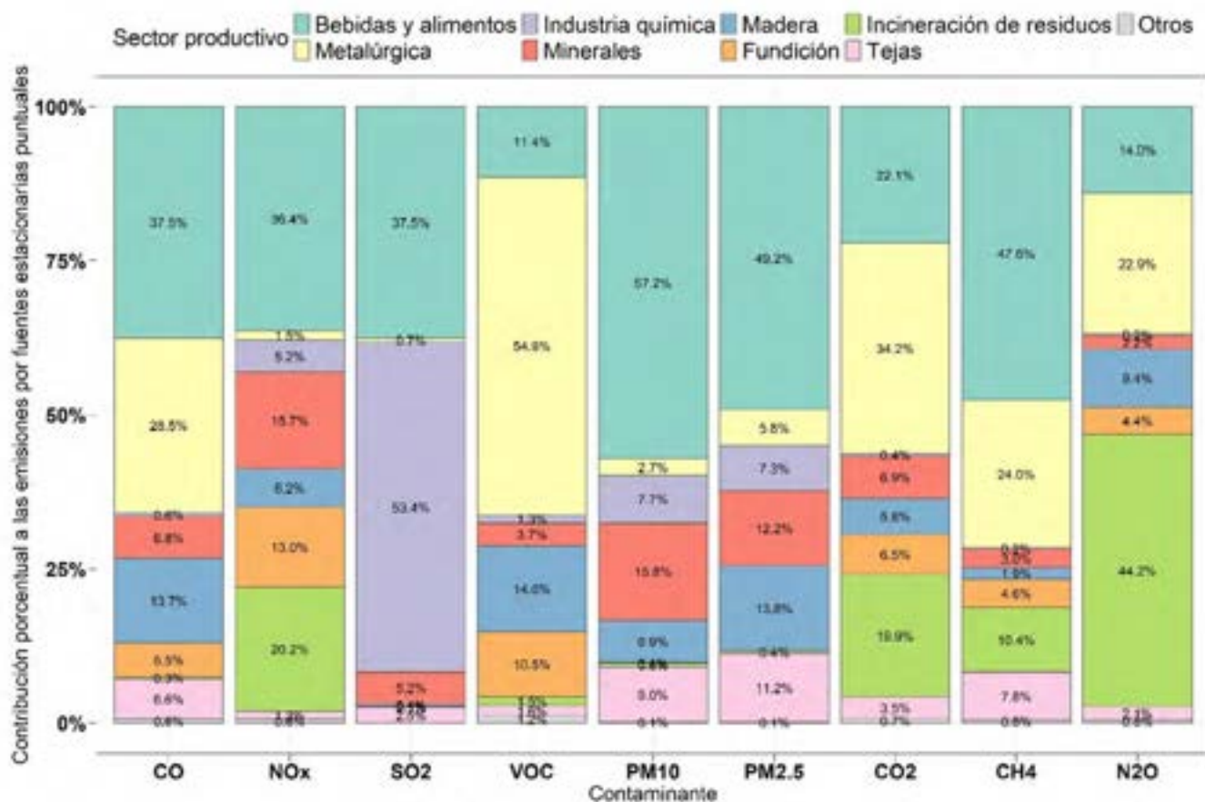
Figura 1. Aporte porcentual del tipo de industria al total de emisiones por fuentes estacionarias puntuales Fuente: elaboración propia.
