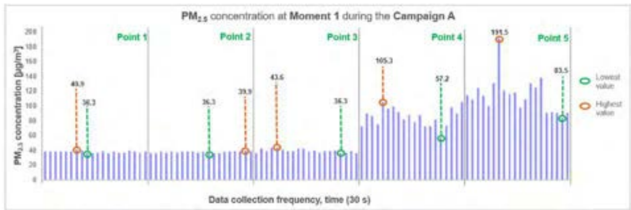
Figura 6. Concentración de PM_{2.5} en el momento 1 de la toma de datos (A). Fuente: Elaboración propia.
