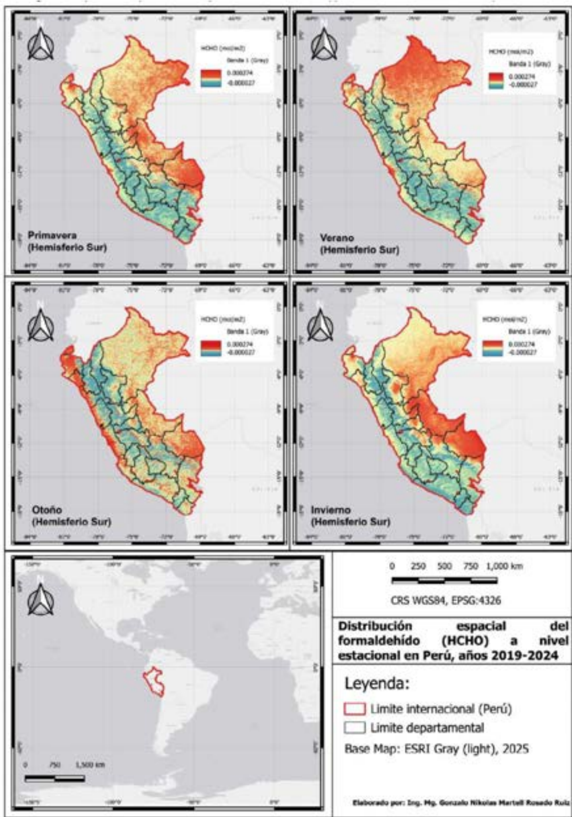
Figura 9. Mapas del comportamiento espacial del HCHO en el Perú, promedios estacionales en mol/m 2 , 2019 al 2024
