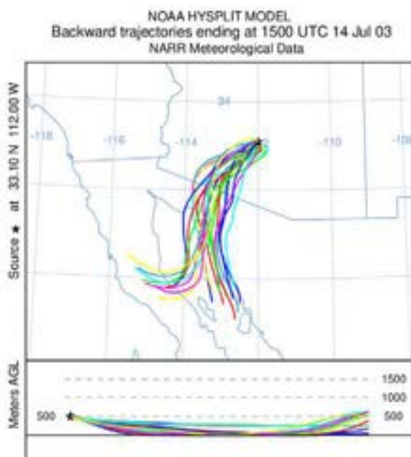
Figura 2. Retrotrayectorias de Hysplit a) Maricopa en Julio del 2003 y b) Tucson en Septiembre del 2020. Fuente: Elaboración propia.
