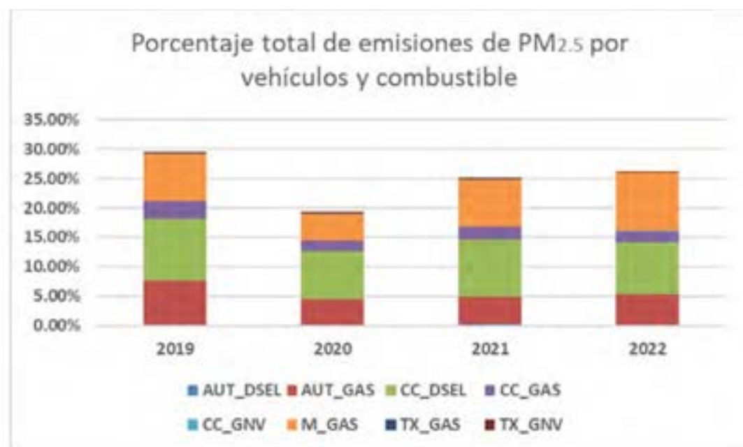
Figura 1: Evolución de las emisiones de PM 2.5 en los años 2019, 2020, 2021 y 2022, categorizada por tipo de vehículos y combustible.
