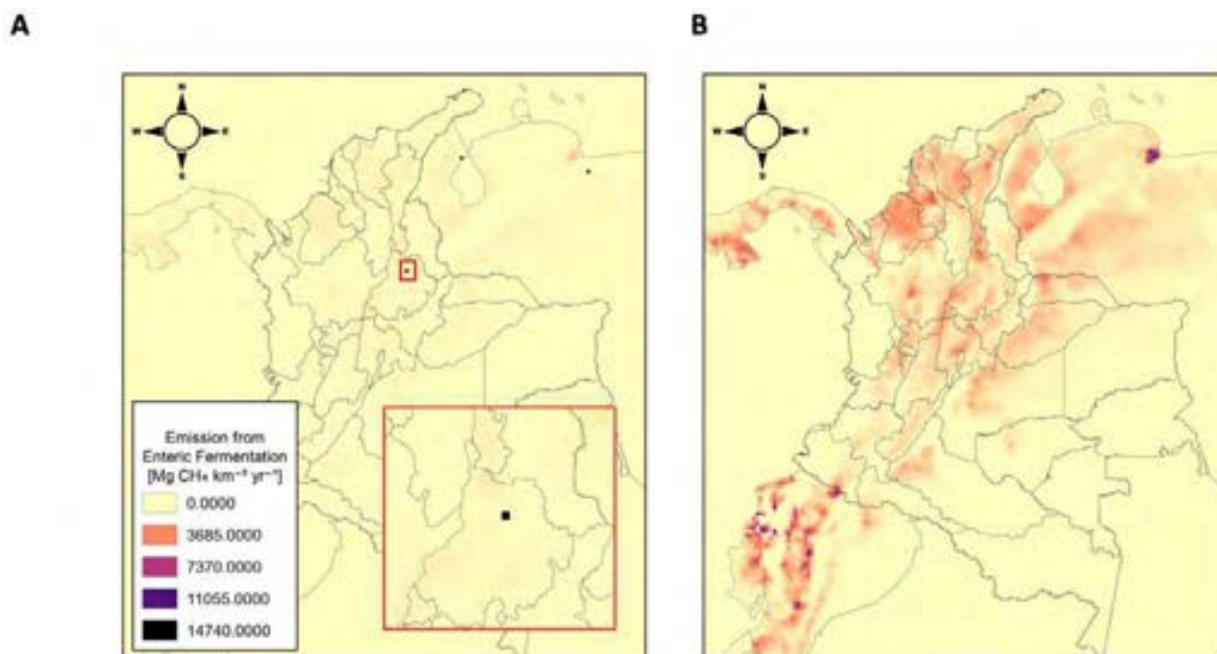
Figura 1. Identificación y eliminación de datos atípicos para fermentación entérica en la base de datos EDGAR v8 GHG 2022. A). Base de datos sin depurar. B). Base de datos depurada.
