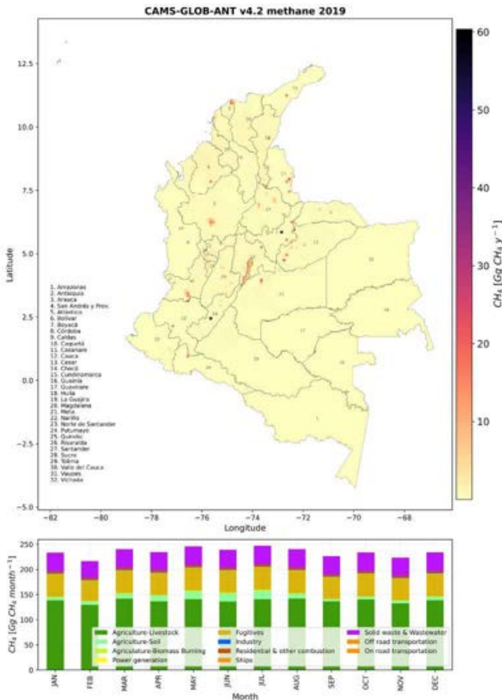
Figura 2. Distribución espacial y temporal de emisiones de metano según la base de datos CAMS-GLOB ANT v4.2 2019. Fuente: Elaboración propia.
