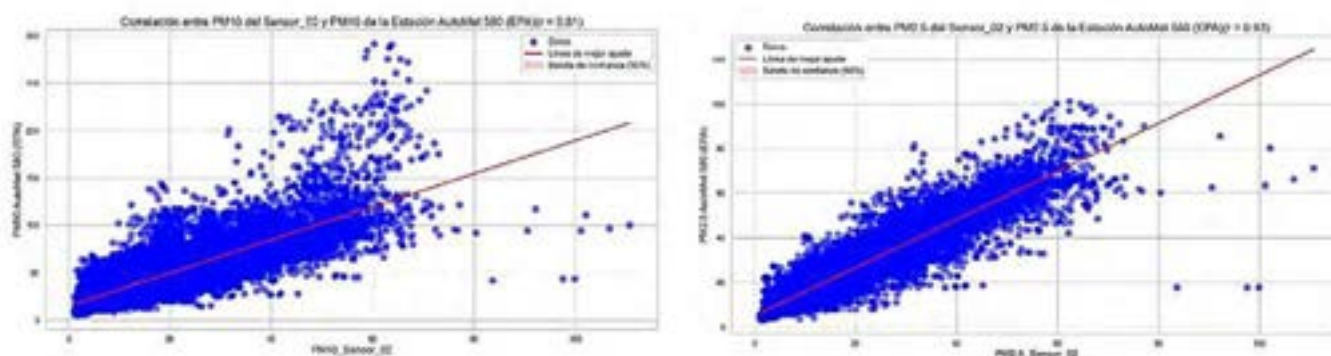
Figura 4. Correlación Sensor 02 SPS-30 vs. Estación EPA (PM2.5 - PM10, Bogotá 2024-2025). Fuente: Autores (2025).
