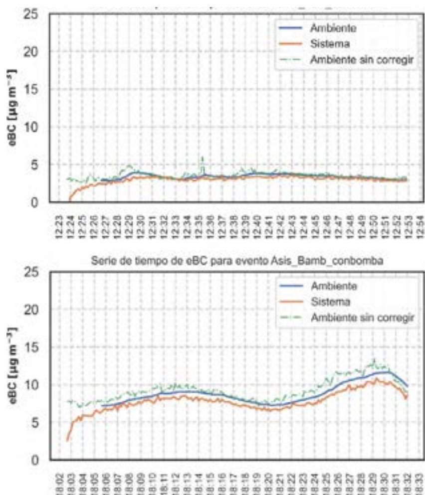
Figura 6. Pruebas de pérdidas de partículas de BC en el sistema. Un microaethalómetro mide la concentración directamente (Ambiente) mientras el otro microaethalómetro se acopla al montaje (Sistema). Se realizaron dos configuraciones, en la configuración B se intercambian los microaethalómetros de la configuración A, es decir, el equipo que medía concentración ambiente en A ahora se acopla al sistema para la configuración B mientras que el equipo midiendo en sistema en la configuración A ahora mide en el ambiente directamente.
