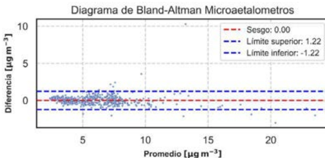
Figura 3. Diagrama de Bland-Altman para mediciones simultáneas de eBC con microaetalómetros de la misma referencia con una resolución temporal de 10 segundos. Fuente: Elaboración propia.
