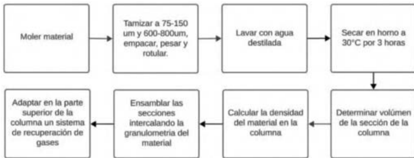
Figura 1. Preparación del eco material y ensamblaje de la columna. Fuente: Autoría propia, 2025.
