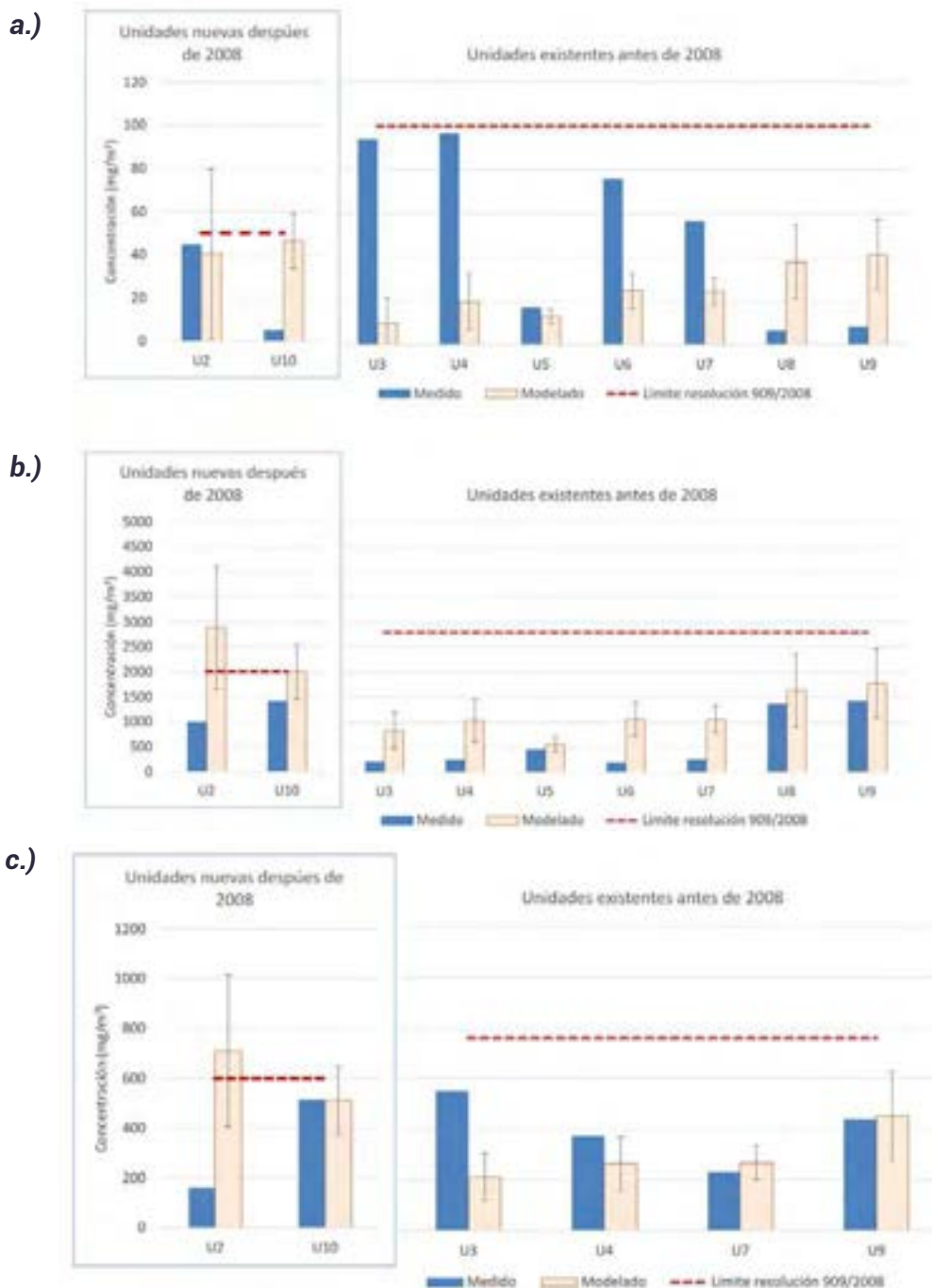
Figura 2. Comparación de concentraciones de emisiones modeladas y mediciones reportadas para las unidades a termoeléctricas a carbón en 2022 a) PST, b) SO 2 y c) NO x . El intervalo, representado por las barras negras, indica la desviación estándar de los datos modelados.
