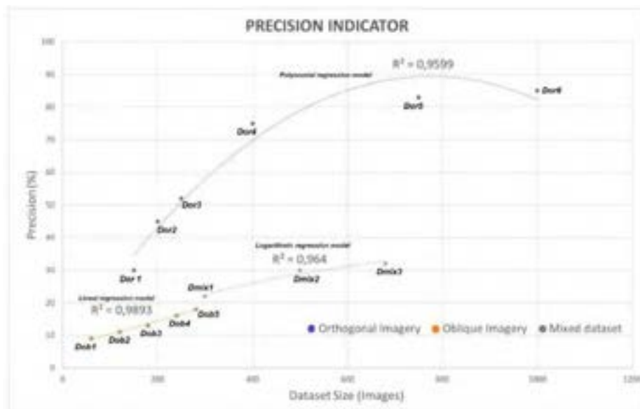
Figura 3. Resultados del indicador Precision para cada dataset. Fuente: Elaboración propia.
