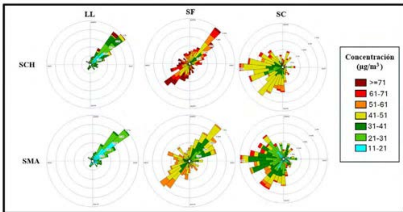
Figura 1. Rosa de concentración de PM_{2.5} .
