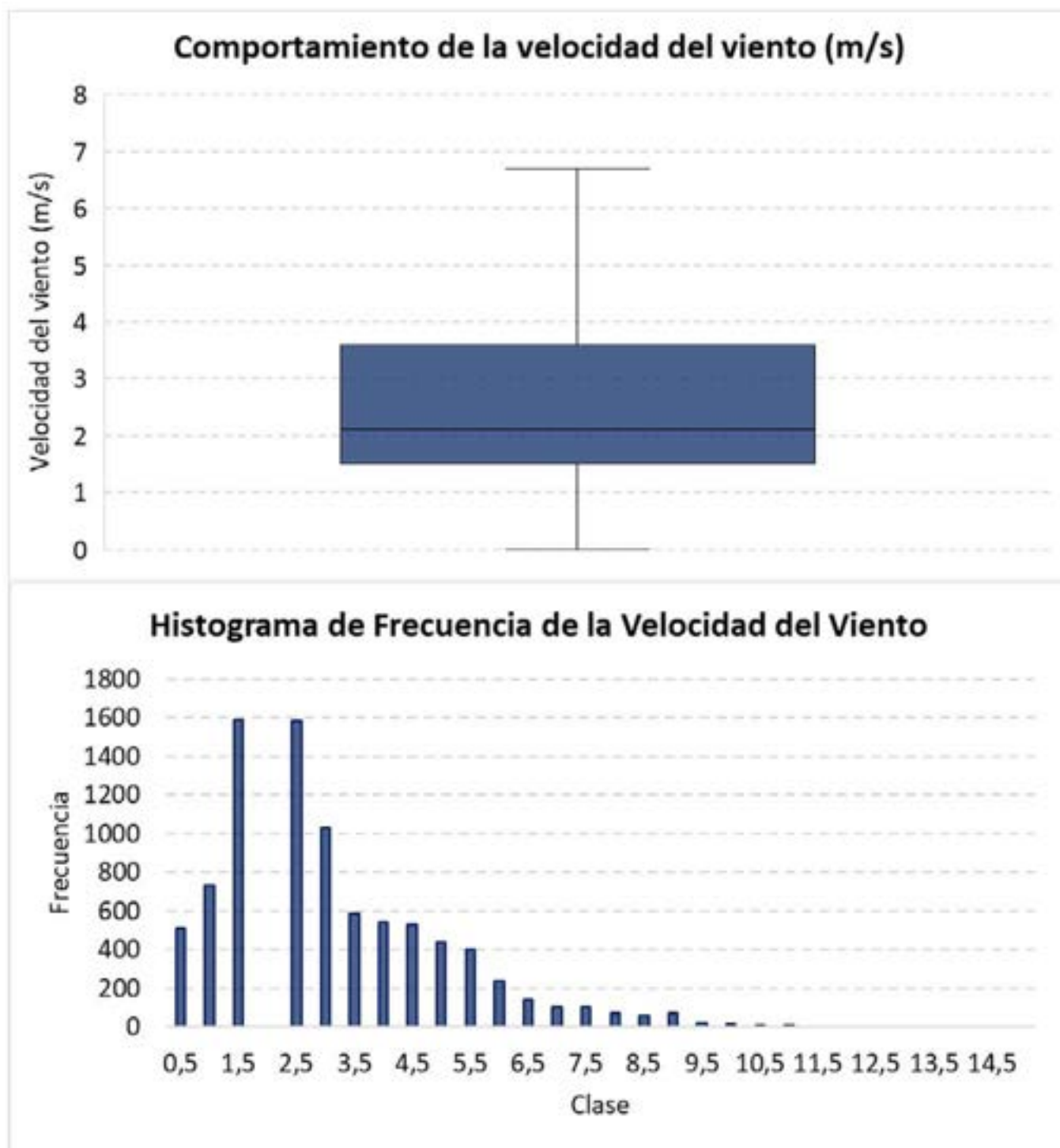
Figura 1 Diagrama de cajas y bigotes e histograma de frecuencia para la velocidad del viento – WRF 2023. Fuente: EYC GLOBAL 2024
