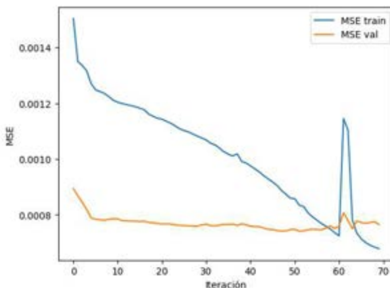
Figura 4. Resultados de rendimiento, evaluados con MSE de un modelo LSTM (Fuente propia).
