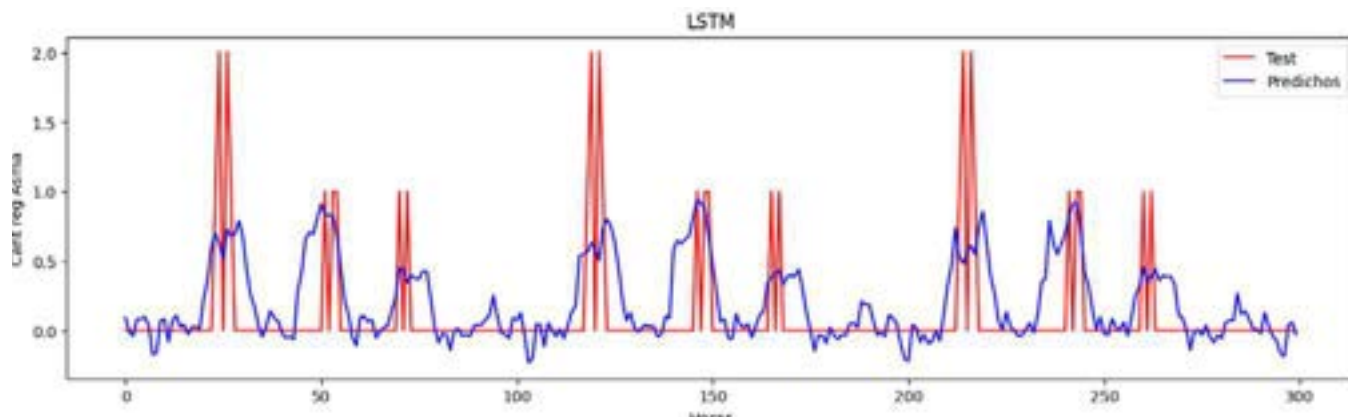
Figura 5. Valores de validación vs valores predichos por el modelo LSTM (Fuente propia).
