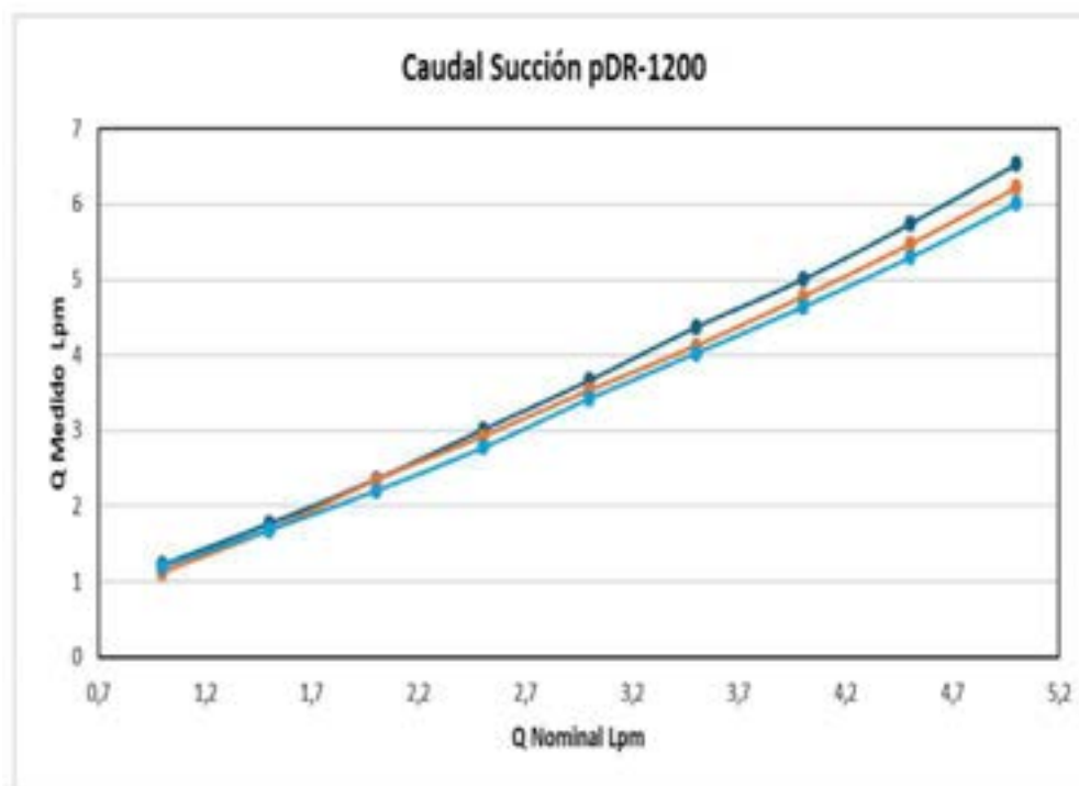
Figura 1. Curva de calibración de caudal
