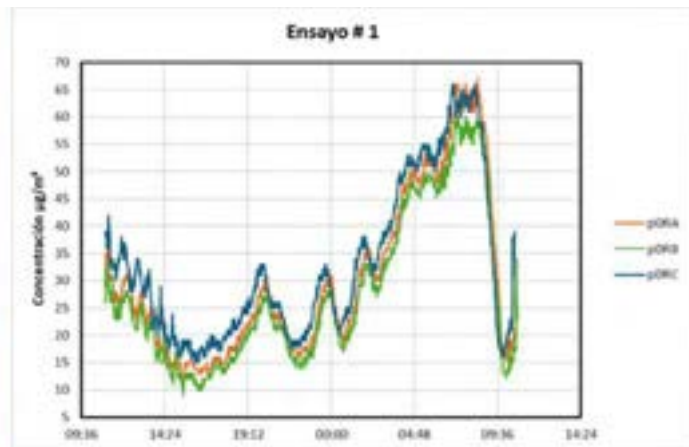
Figura 2. Concentraciones medidas por los Pdr-1200.
