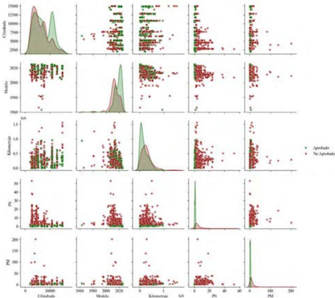
Figura 8. Relación entre variables técnicas del vehículo y emisiones de PN y PM. Fuente: Elaboración propia
